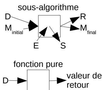
FIGURE 7 – Spécification d'une procédure. D : arguments données, E : entrées directes (lectures dans un fichier, dans le corps du sous-algorithme), R : arguments résultats, S : écritures directes (écritures dans un fichier, dans le corps du sous-algorithme), M : arguments données-résultats. La spécification d'un sous-algorithme indique comment (R, M_{\text{final}} , S) dépend de (D, M_{\text{initial}} , E). La spécification d'une fonction pure indique comment la valeur de retour dépend de D.
