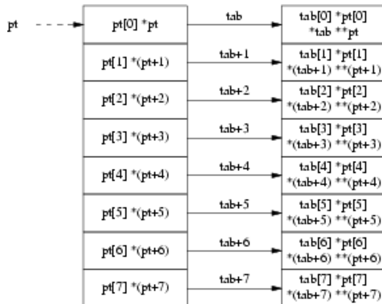
FIG. 10.6 – Tableau de pointeurs sur des variables dans un tableau
