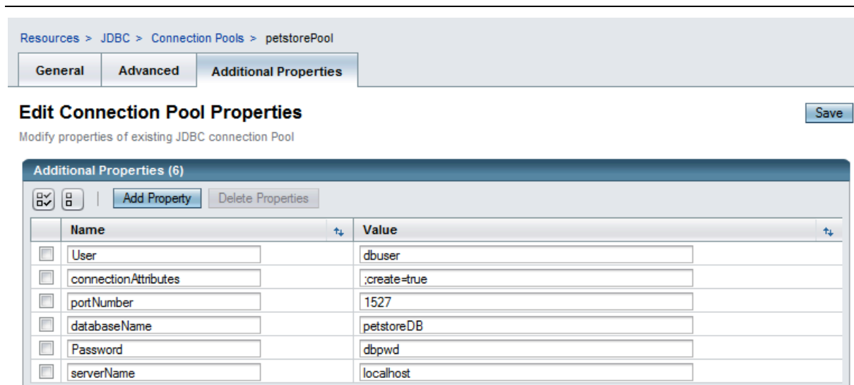
Figure 5-5: Propriétés du pool de connexion
