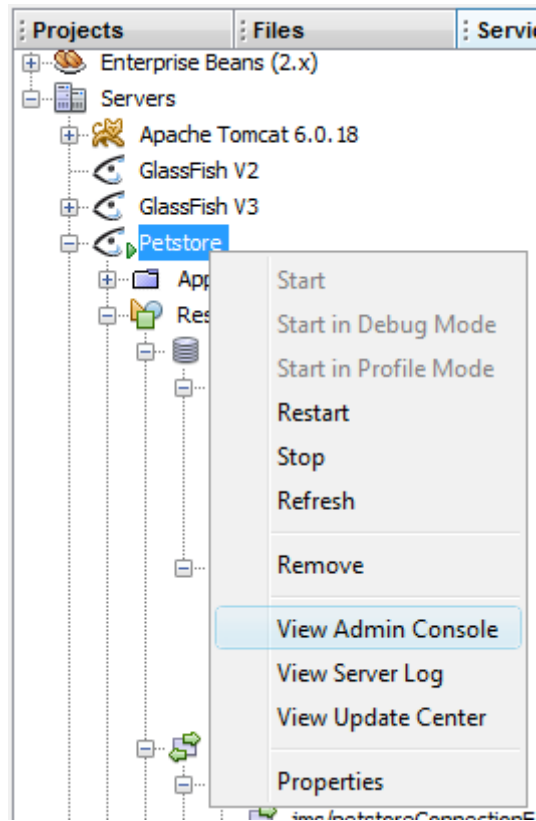
Figure 6-12: Accès à la console d'administration
