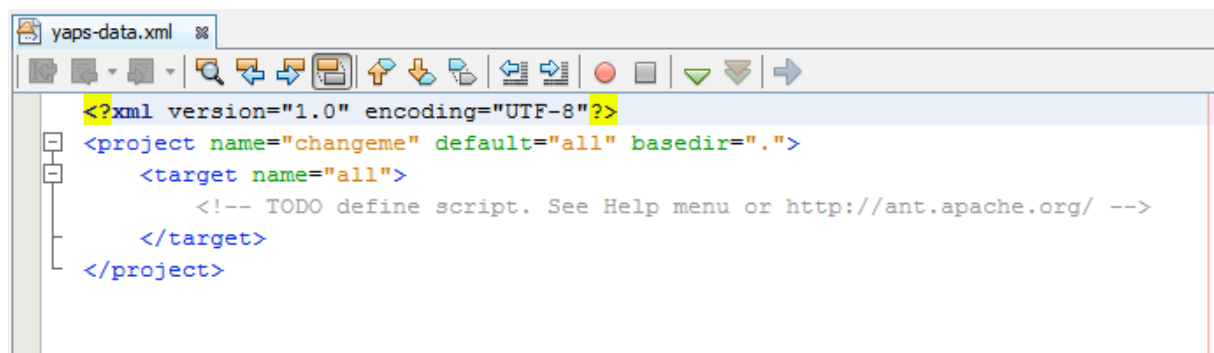
Figure 9-44: Fichier yaps-data.xml
