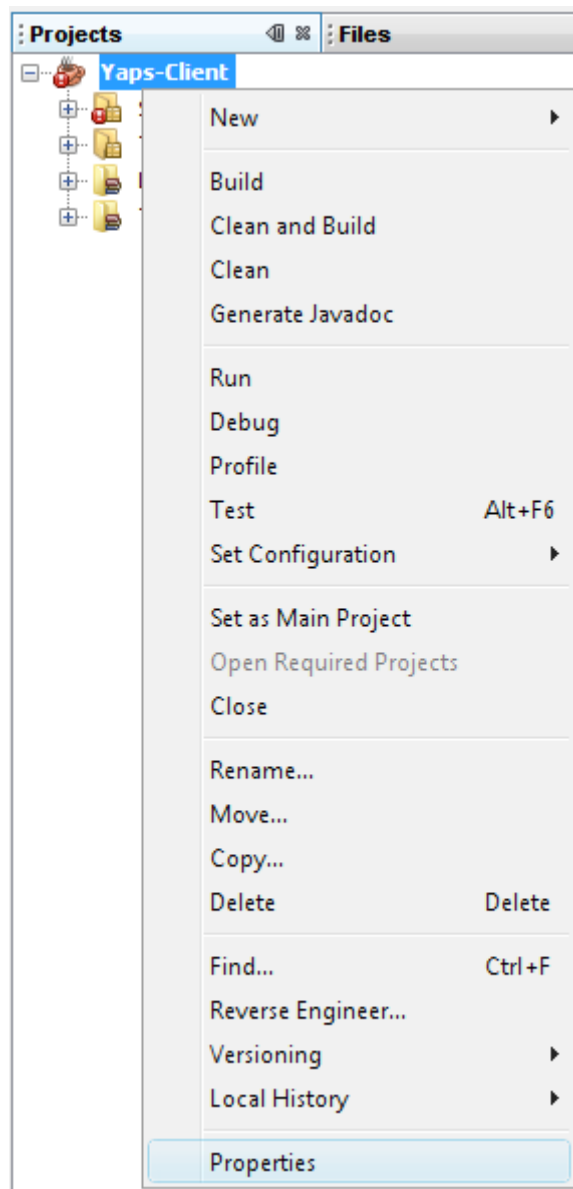
Figure 10-6: Menu propriétés
