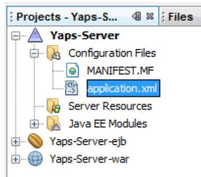
Figure 9-21: Fichier « application.xml »
