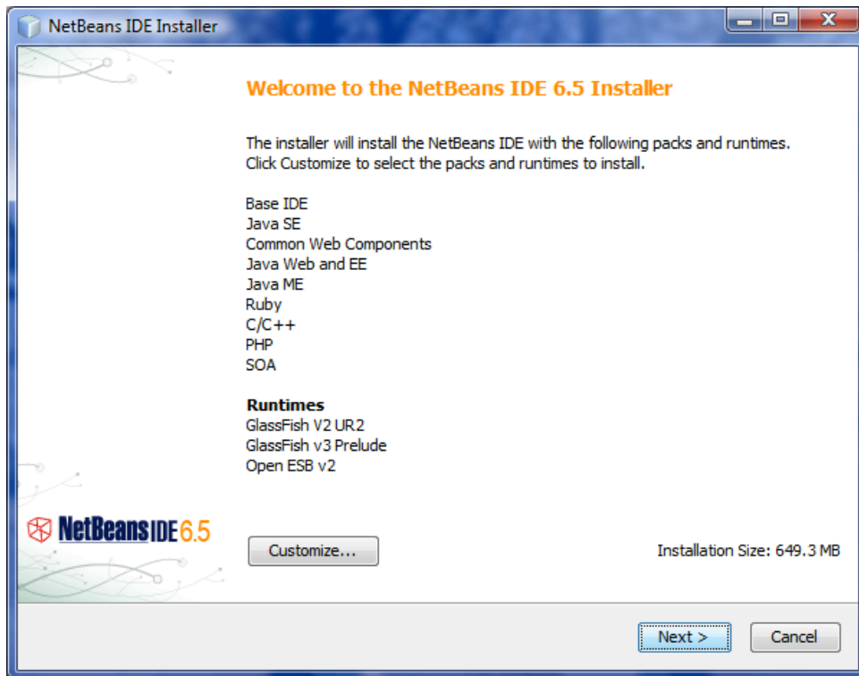
Figure 3-4: Page d'accueil
