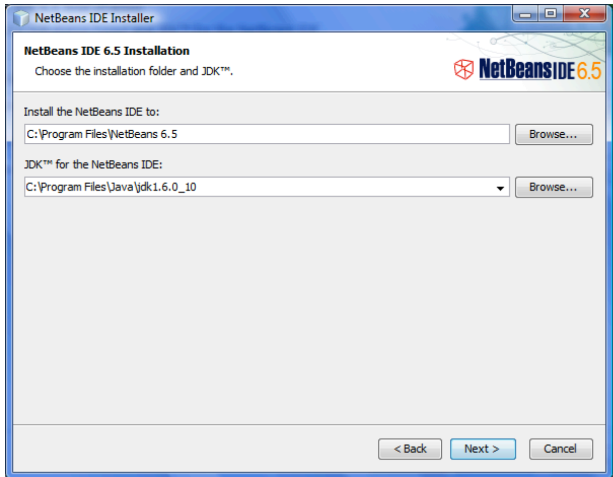
Figure 3-7: Répertoires d'installation
