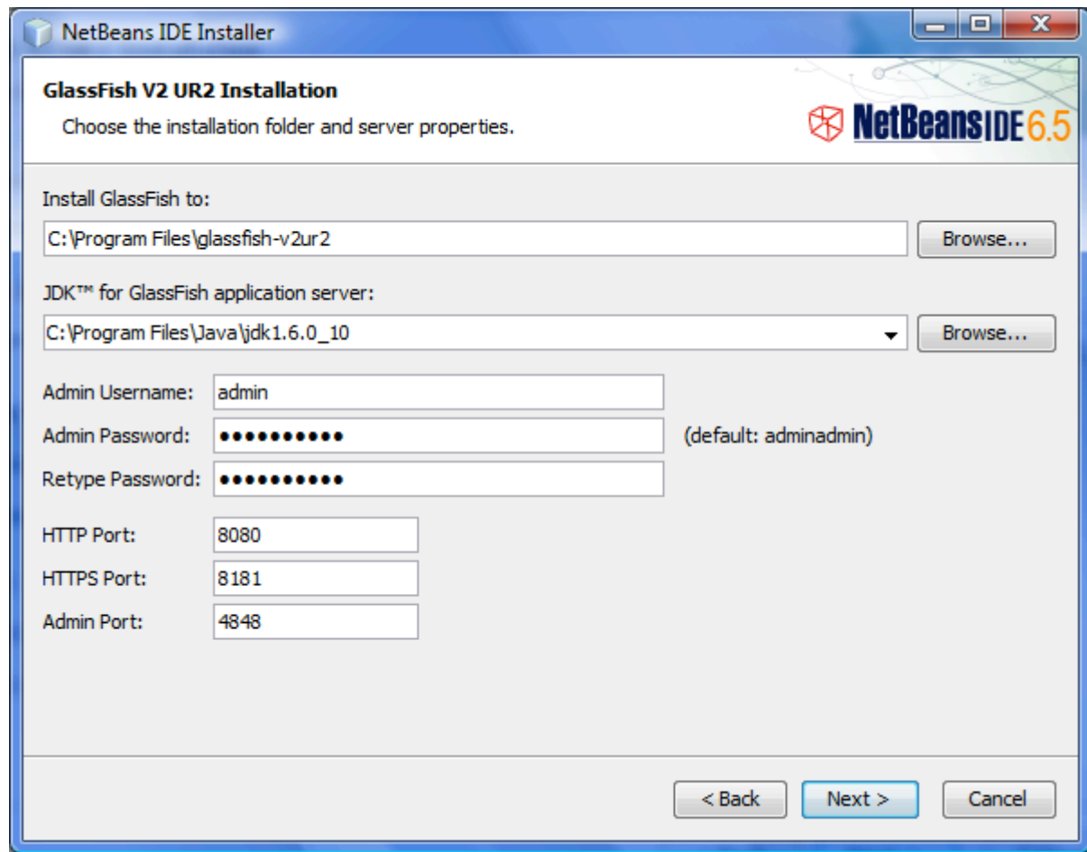
Figure 3-8: Paramètres de GlassFish V2
