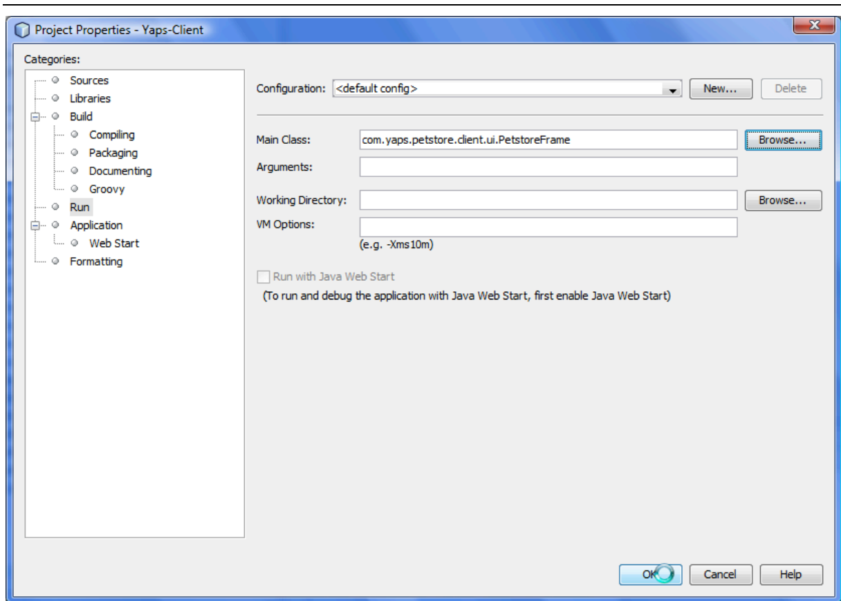
Figure 10-24: Classe principale identifiée
