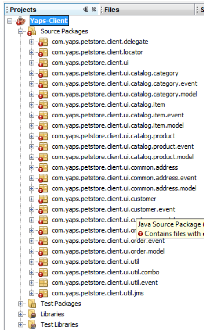
Figure 10-5: Projet Yaps-Client après le transfert
