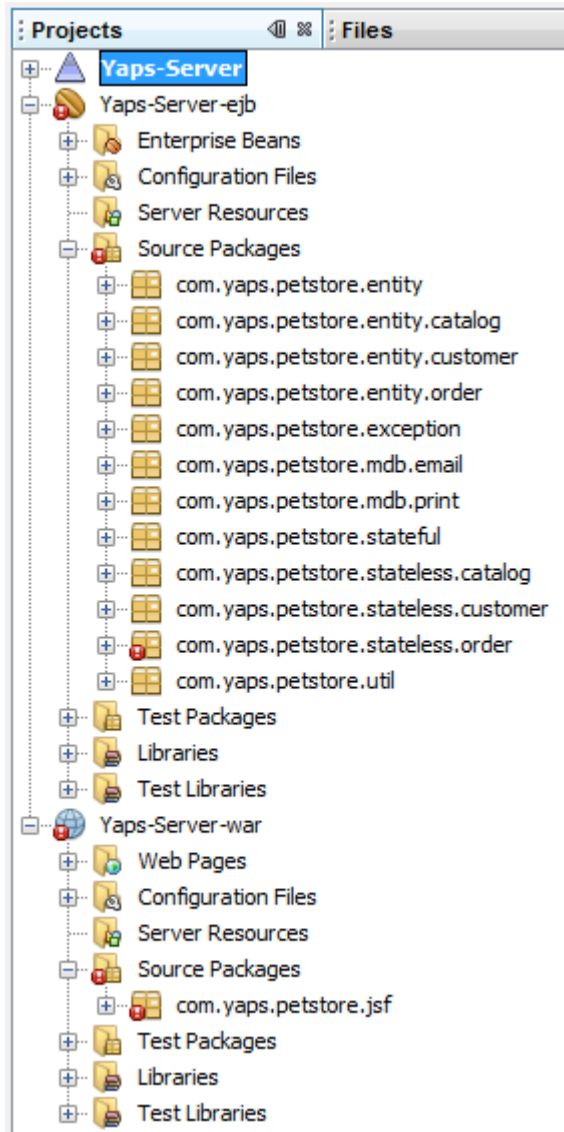
Figure 9-6: Projet Yaps-Server après le transfert
