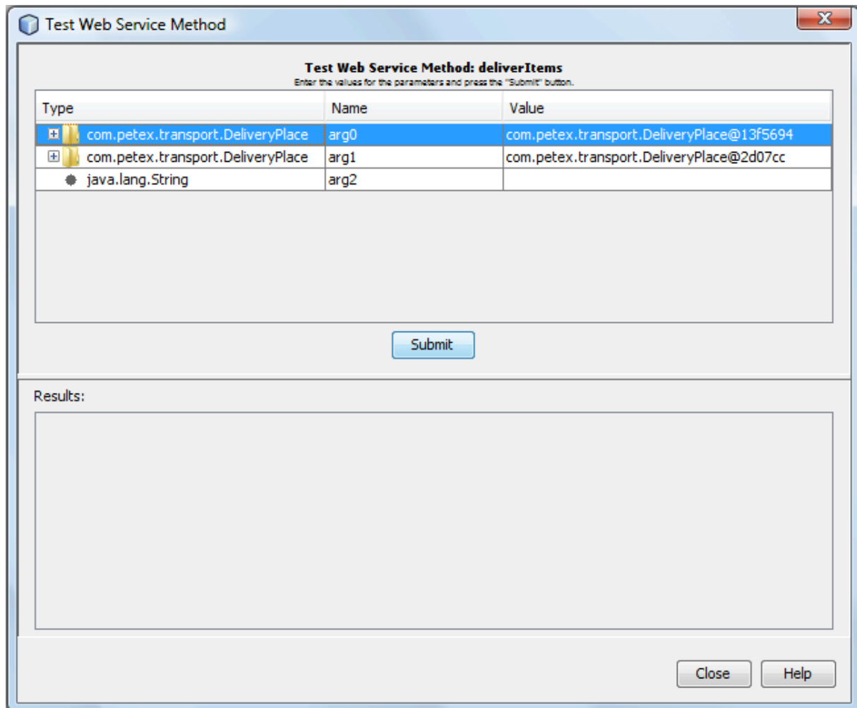
Figure 8-20: Écran de test du Web Service
