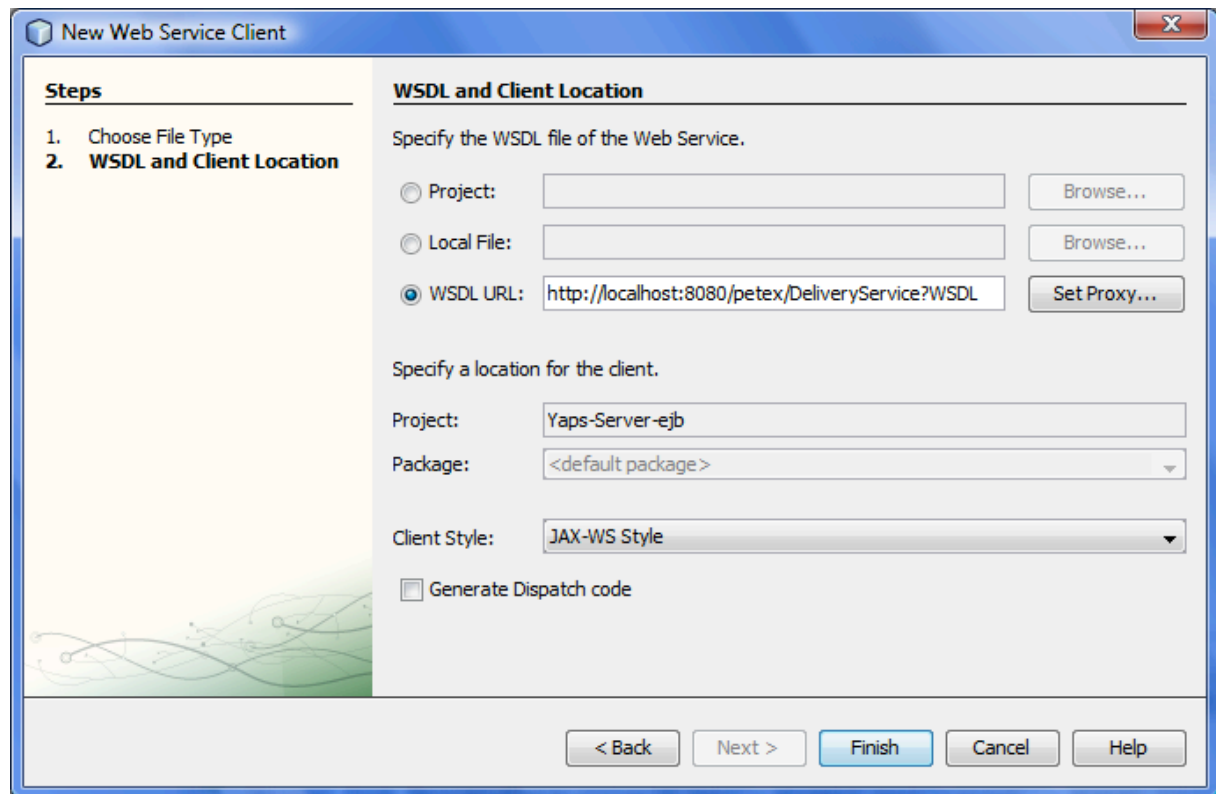
Figure 9-10: Localisation du WSDL
