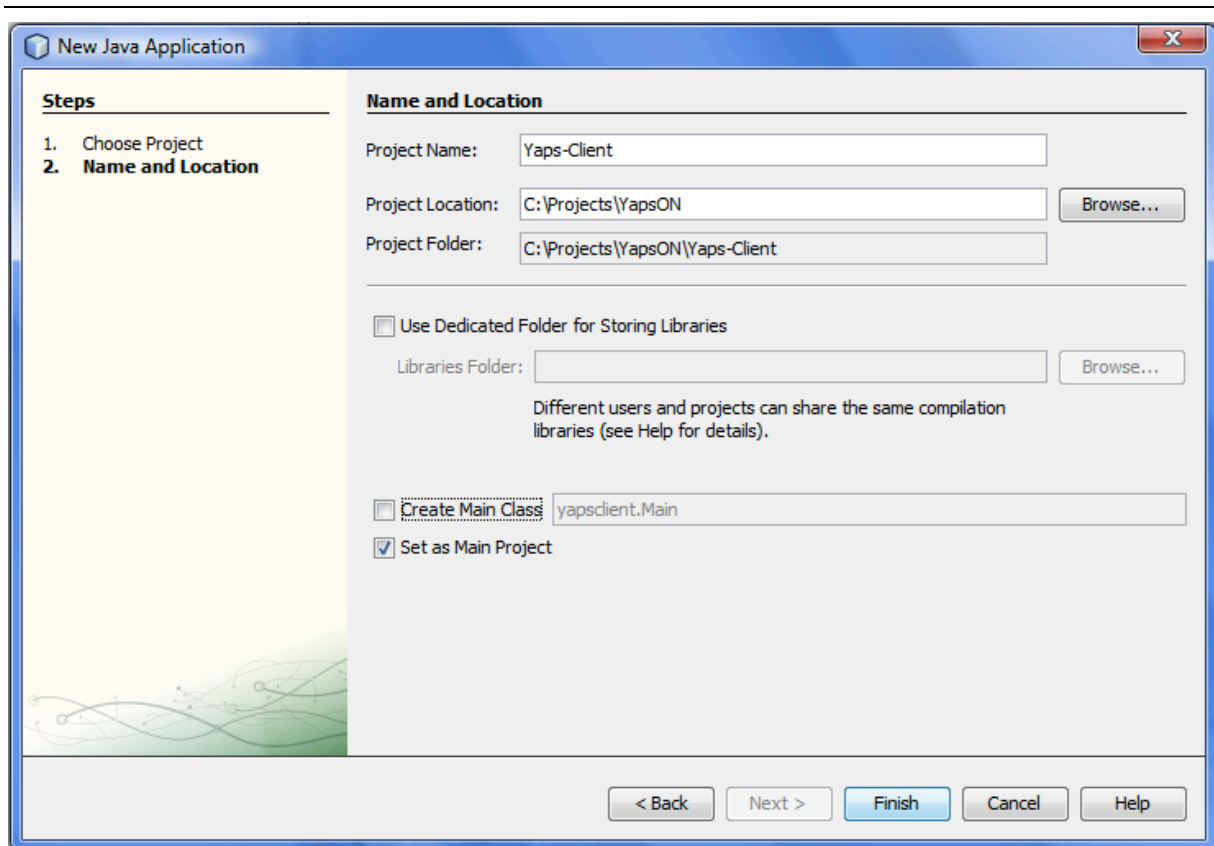
Figure 10-3: Nom du projet et répertoire
