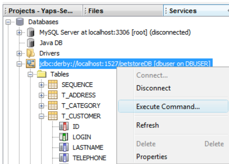
Figure 9-36: Exécuter une commande SQL
