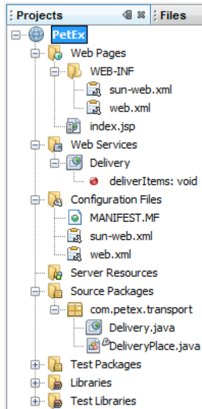
Figure 8-7: Projet PetEx après le transfert
