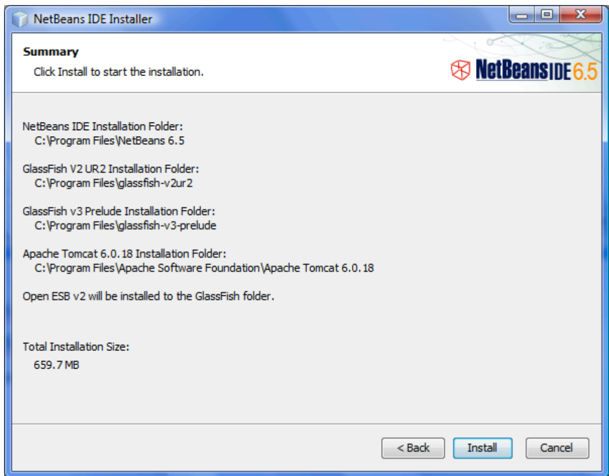
Figure 3-11: Résumé d'installation
