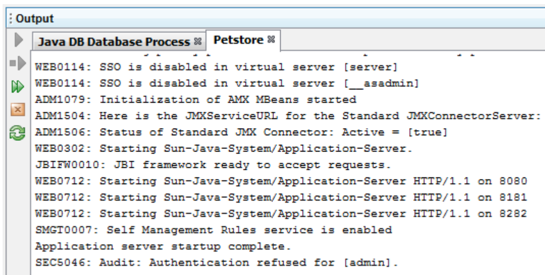
Figure 6-8: Fenêtre "Output"
