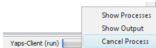
Figure 10-31: Annuler l'exécution
