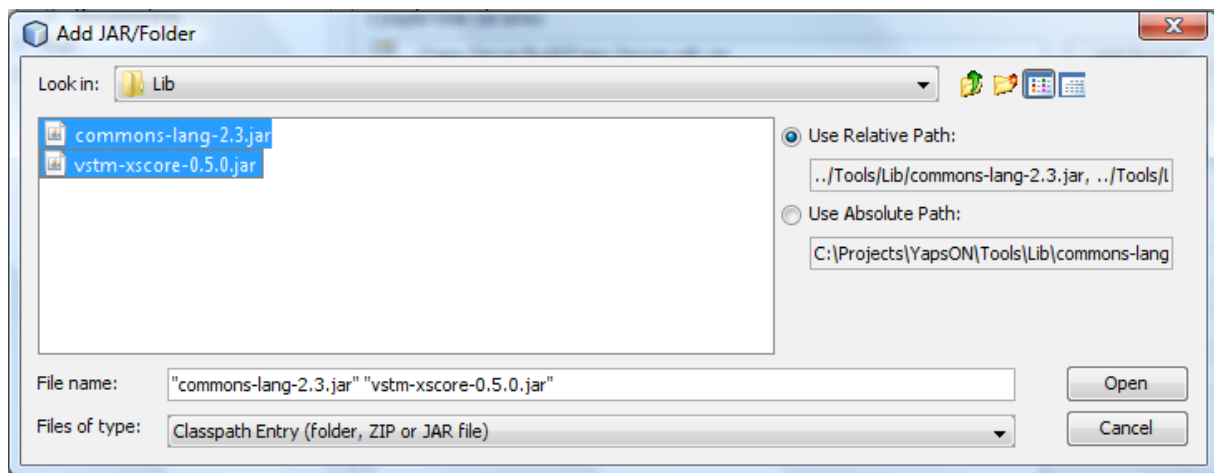
Figure 10-10: Bibliothèques utilitaires
